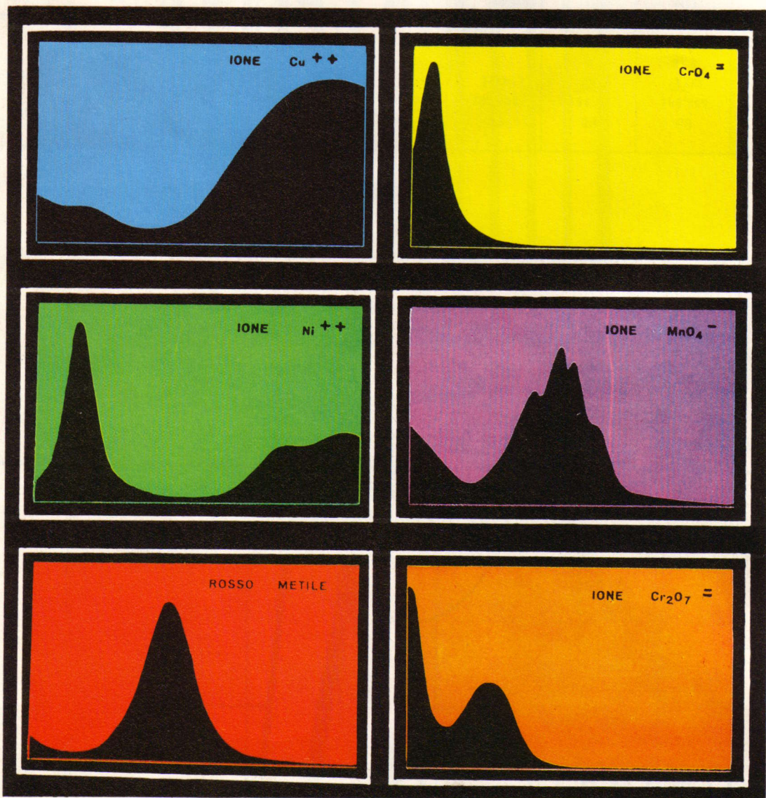
Fig. I, 2 - Colore di alcune sostanze e relativo spettro di assorbimento.
