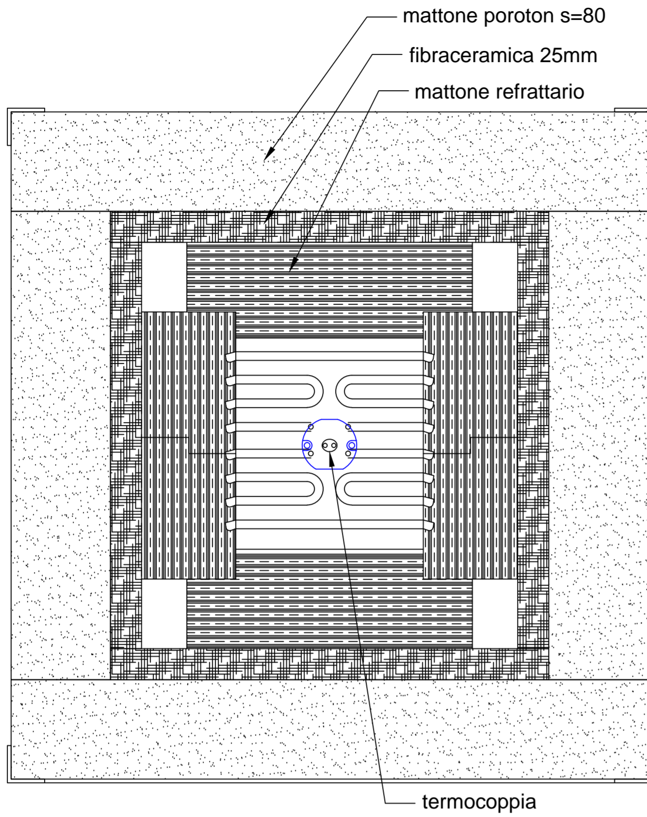
vista frontale
